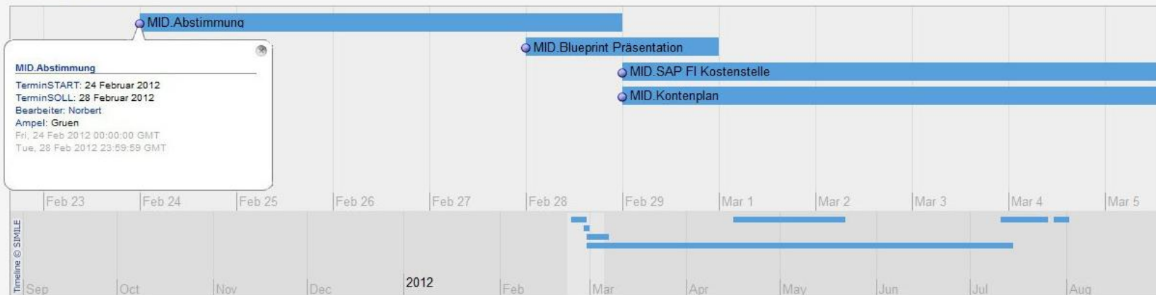
Gantt-Diagramm (generiert)
